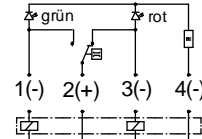
Diode rot/grün Schaltbild 0.347
