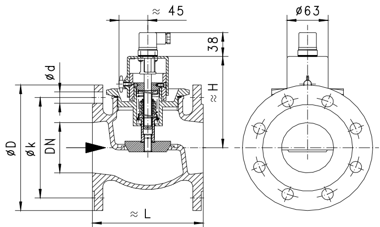
Flanschmaße DIN 2501 PN 16 Dichtleiste DIN 2526 Form C
